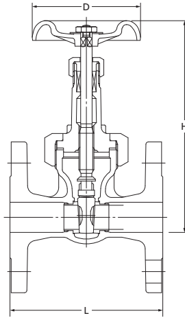
Face to face : JIS B2002 JV 4-2 End connection : JIS B2239 16K
